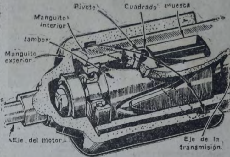
Dibujo en corte de la nueva caja de velocidades mostrando solamente las partes principales del mecanismo interno. La cubierta y la bomba de control de los cuadrados, no aparece en el grabado
